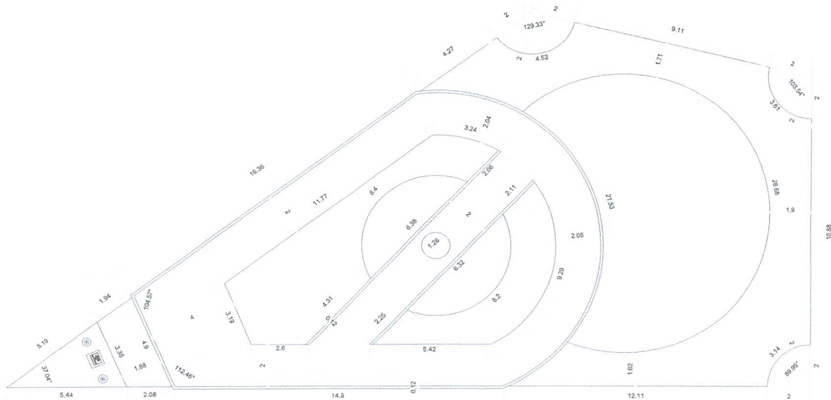
PLANTA DIMENSIONADA DE CONJUNTO PARQUE RANCHO NUEVO Escala: 1:100
