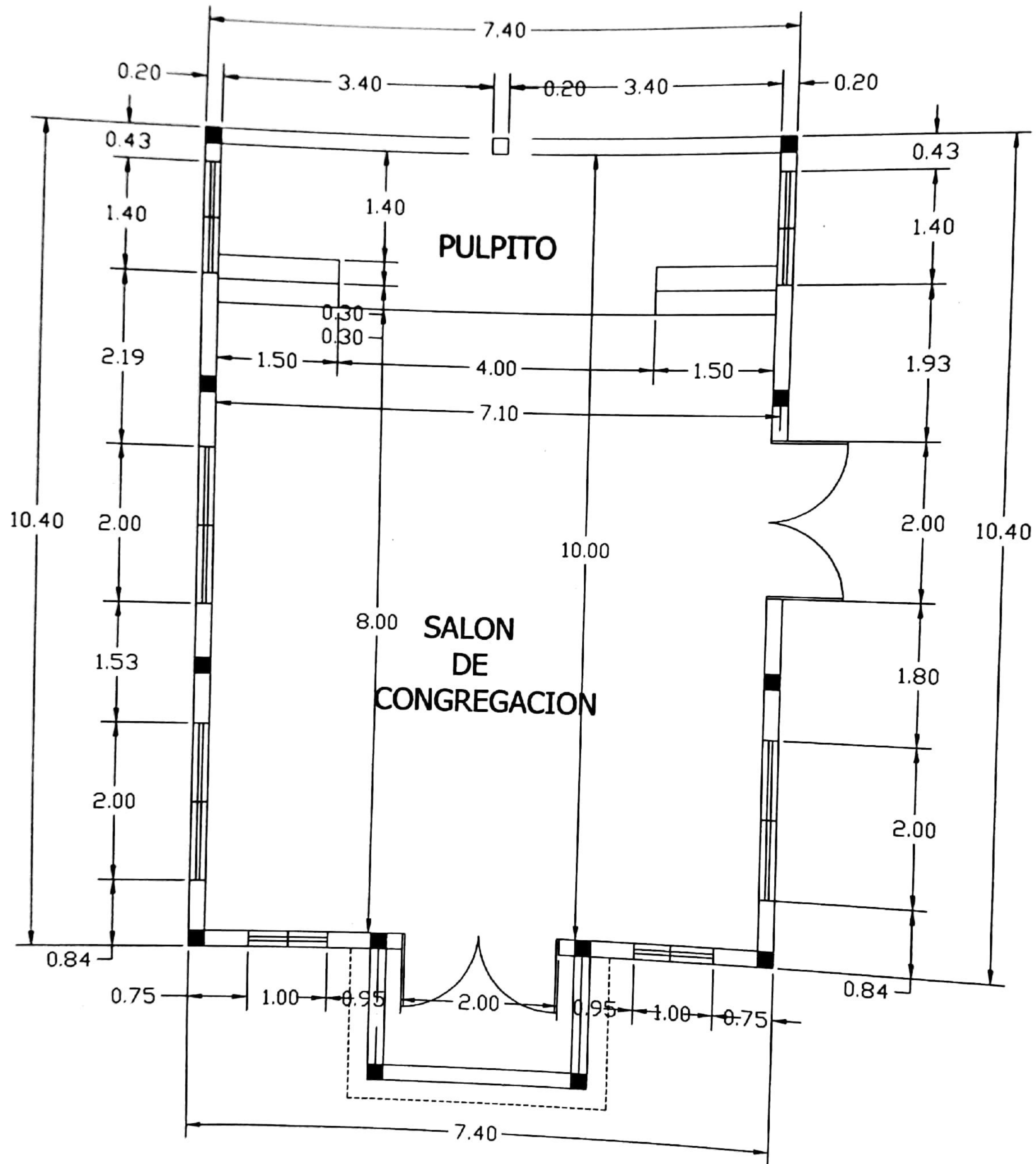
PLANTA DIMENSIONADA
