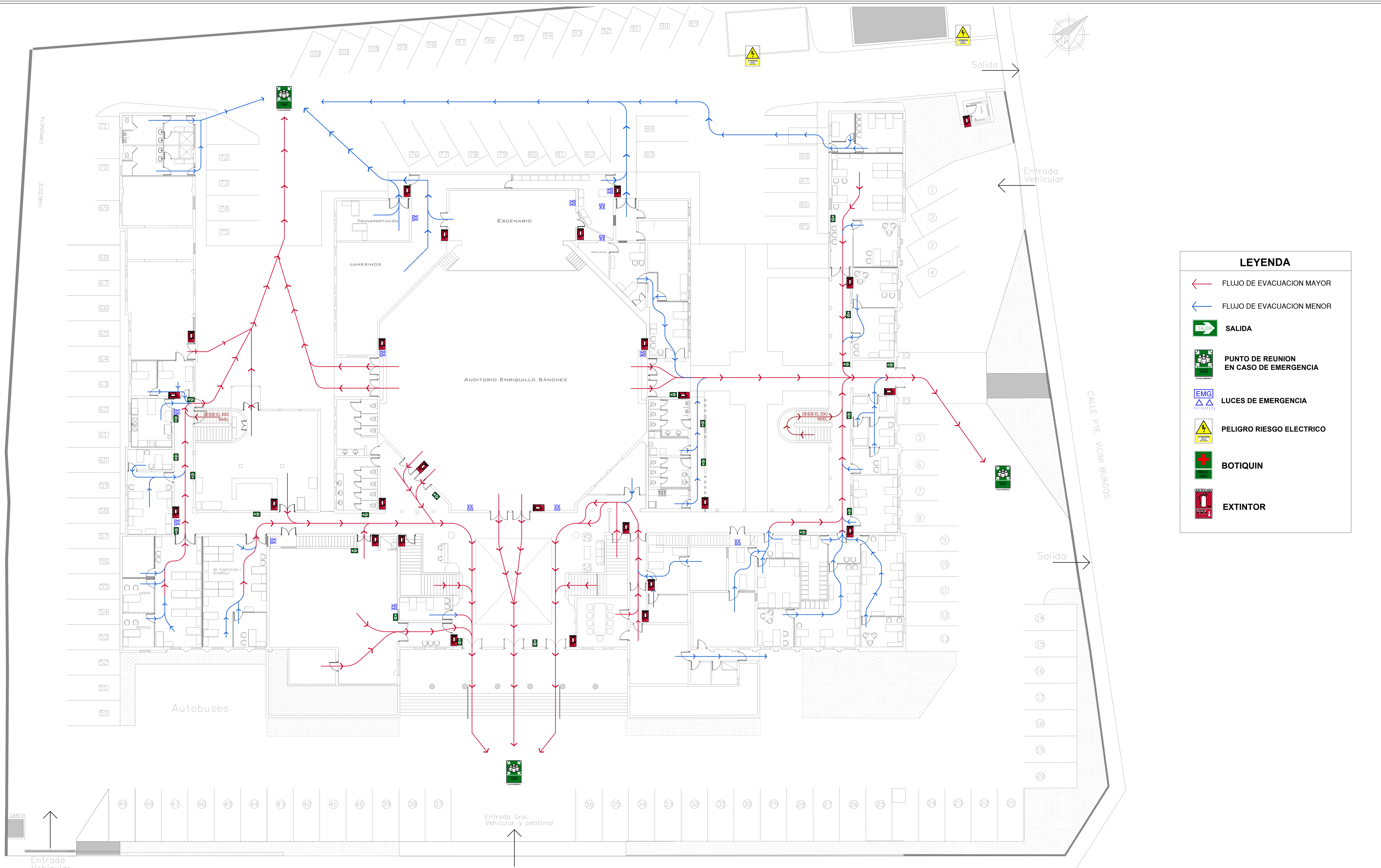
PLANO RUTA DE EVACUACION_1ER NIVEL SEDE MINC ESC. 1:150 MTS.
