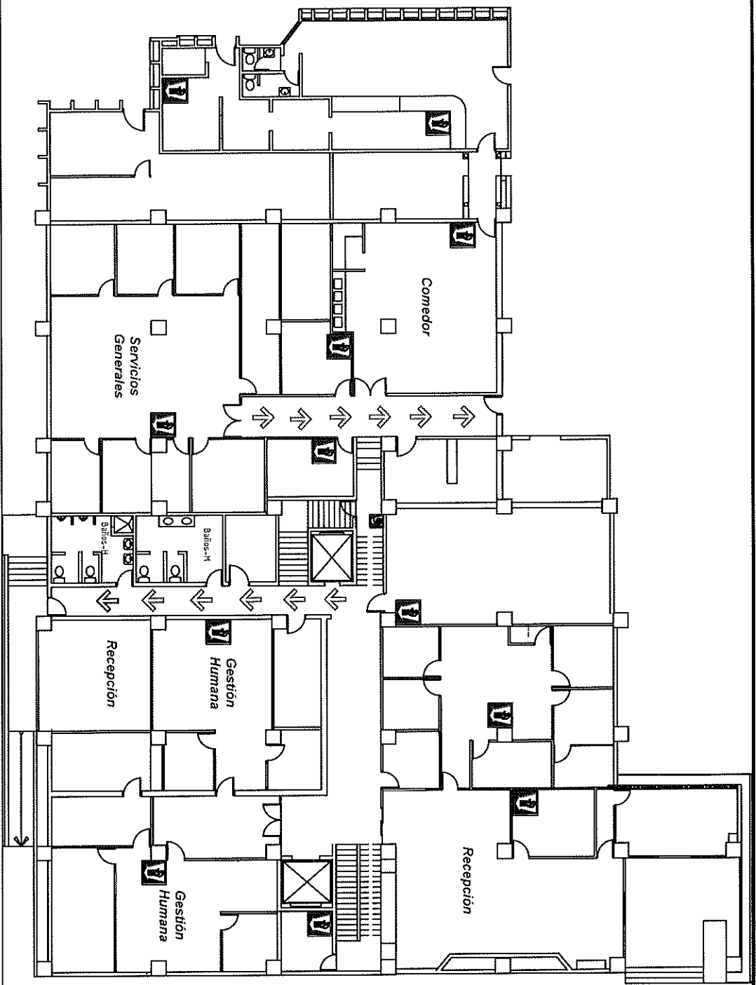
PLANTA ARQUITECTONICA PRIMER NIVEL
